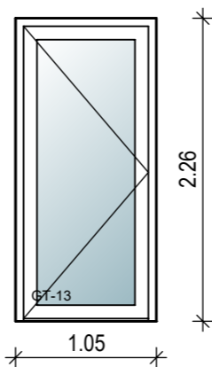
Pos.-Nr. 6.1.1 1-teiliges Tür-Element Notausgang 1,05m x 2,26m (2 Stück)
