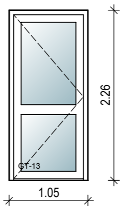
Pos.-Nr. 6.1.4 1-teiliges Tür-Element 1,05m x 2,26m (1 Stück)
