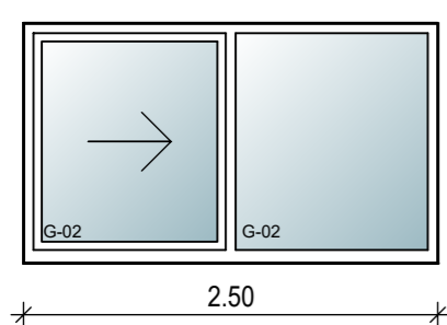
Pos.-Nr. 6.2.11 2-teiliges Schiebe-Fenster-Element 2,50m x 1,45m (1 Stück)
