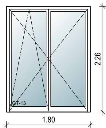
Pos.-Nr. 6.1.1 2-teiliges Fenster-Element 1,80m x 2,26m (12 Stück)
