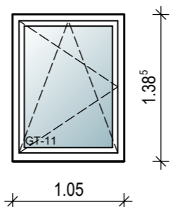
Pos.-Nr. 6.1.3 1-teiliges Fenster-Element 1,05m x 1,385m (3 Stück)
