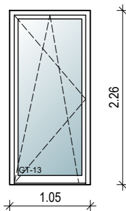
Pos.-Nr. 6.1.2 1-teiliges Fenster-Element 1,05m x 2,26m (2 Stück)
